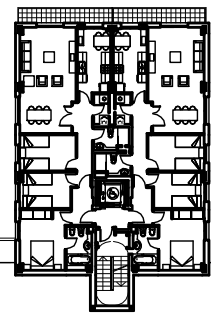
PLANTA TIPO ED.3
