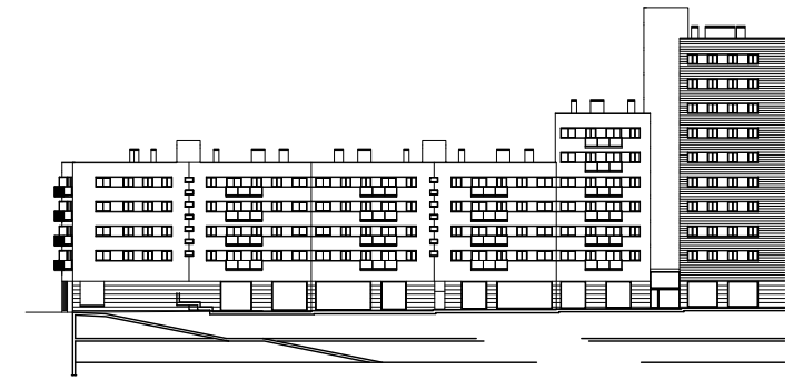
ALZADO ED.2 - PLAZA
