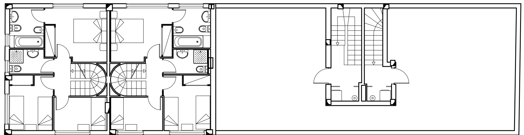
PLANTA SEGUNDA
