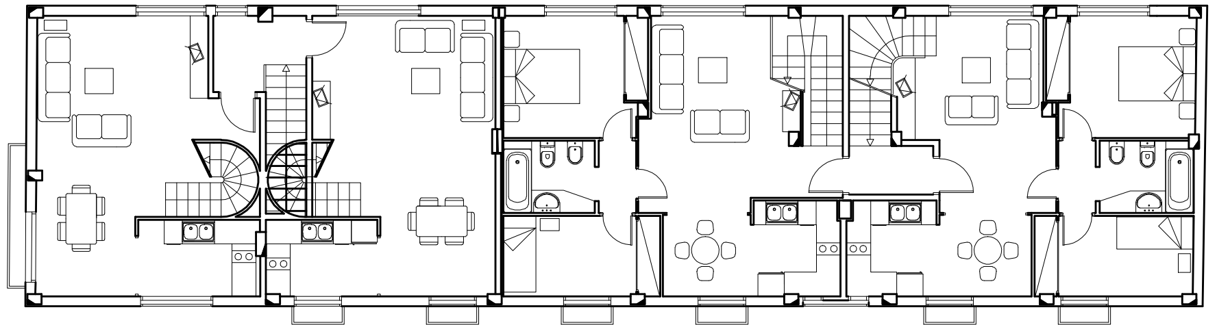
PLANTA PRIMERA
