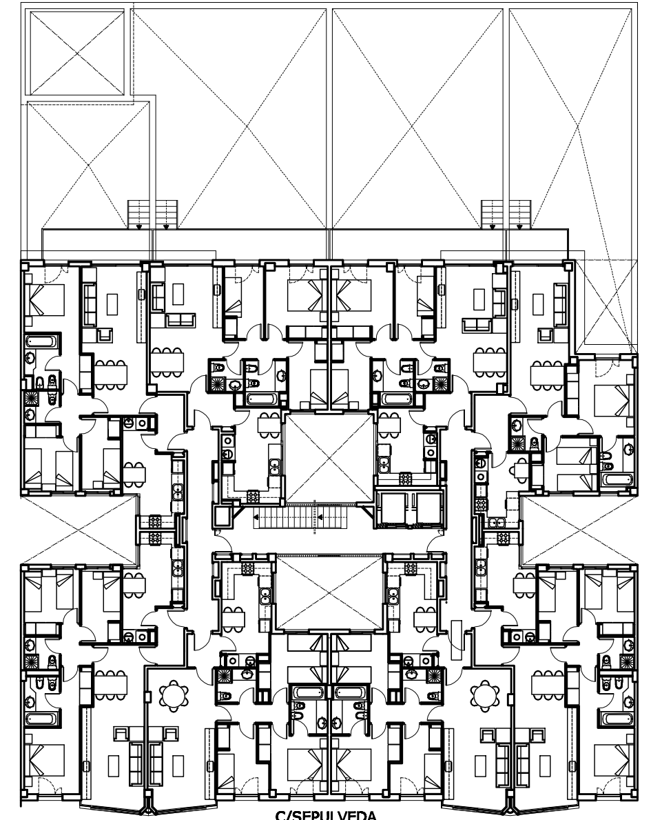
PLANTA PRIMERA
