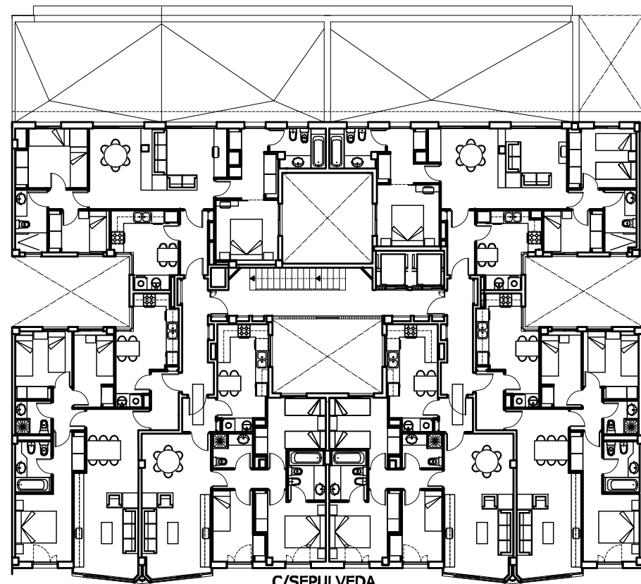
PLANTA TIPO
