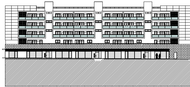
ALZADO BL.1 NORESTE
