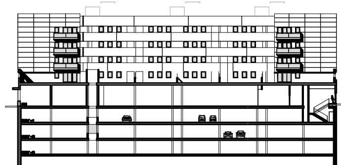
ALZADO BL.1 INTERIOR
