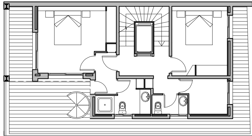
PLANTA SEGUNDA
