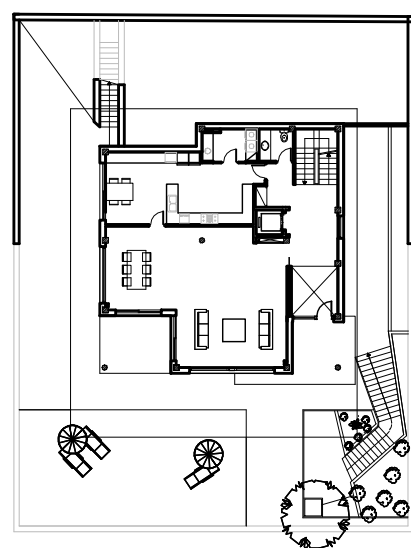
PLANTA BAJA-PARCELA 2
