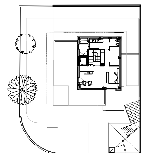
PLANTA SEGUNDA-PARCELA 1
