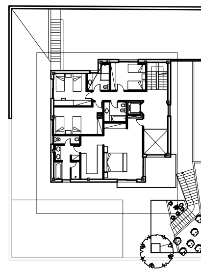
PLANTA PRIMERA-PARCELA 2
