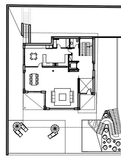
PLANTA BAJA-PARCELA 3
