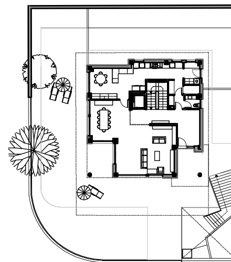
PLANTA BAJA-PARCELA 1
