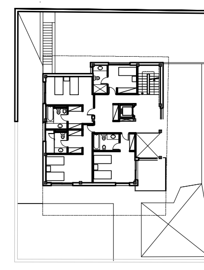
PLANTA PRIMERA-PARCELA 3
