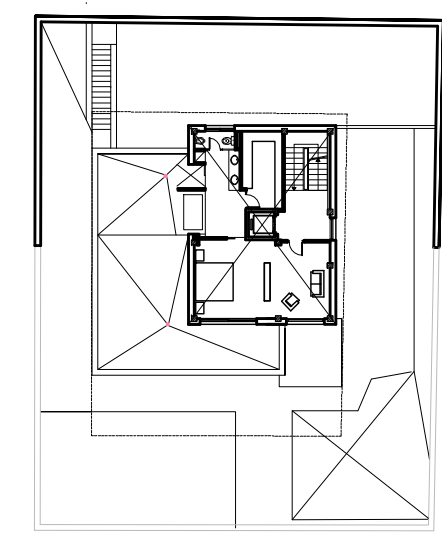
PLANTA SEGUNDA-PARCELA 3
