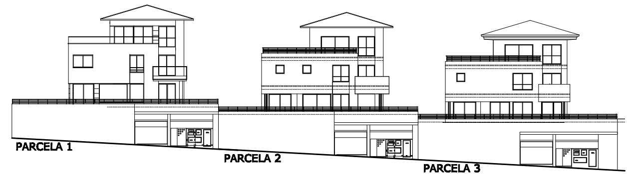
ALZADO VIAL DE NUEVA CREACION
