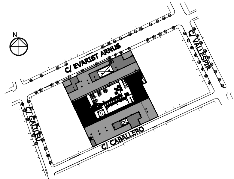
EMPLAZAMIENTO
