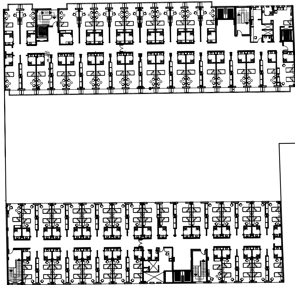
PLANTA PRIMERA
