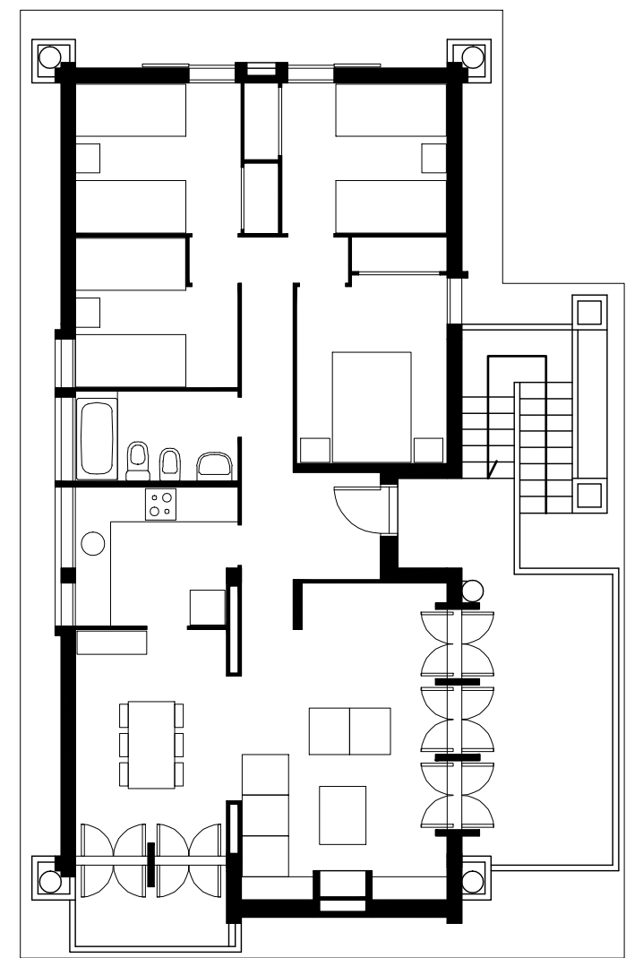
PLANTA PRIMERA
