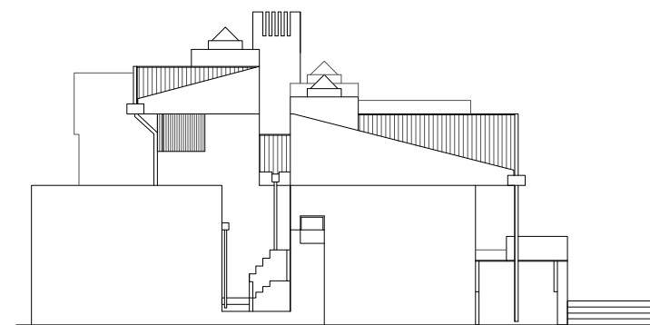
ALZADO SUR
